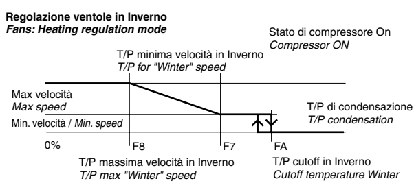
Esempio di F2=3 in modalità Inverno Example of F2=3 Heating mode
