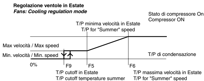
Esempio di F2=3 in modalità Estate Example of F2=3 Cooling mode
